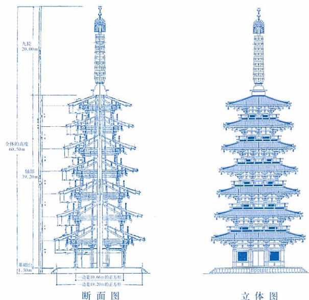
上野国国分寺七层塔复原设计图
